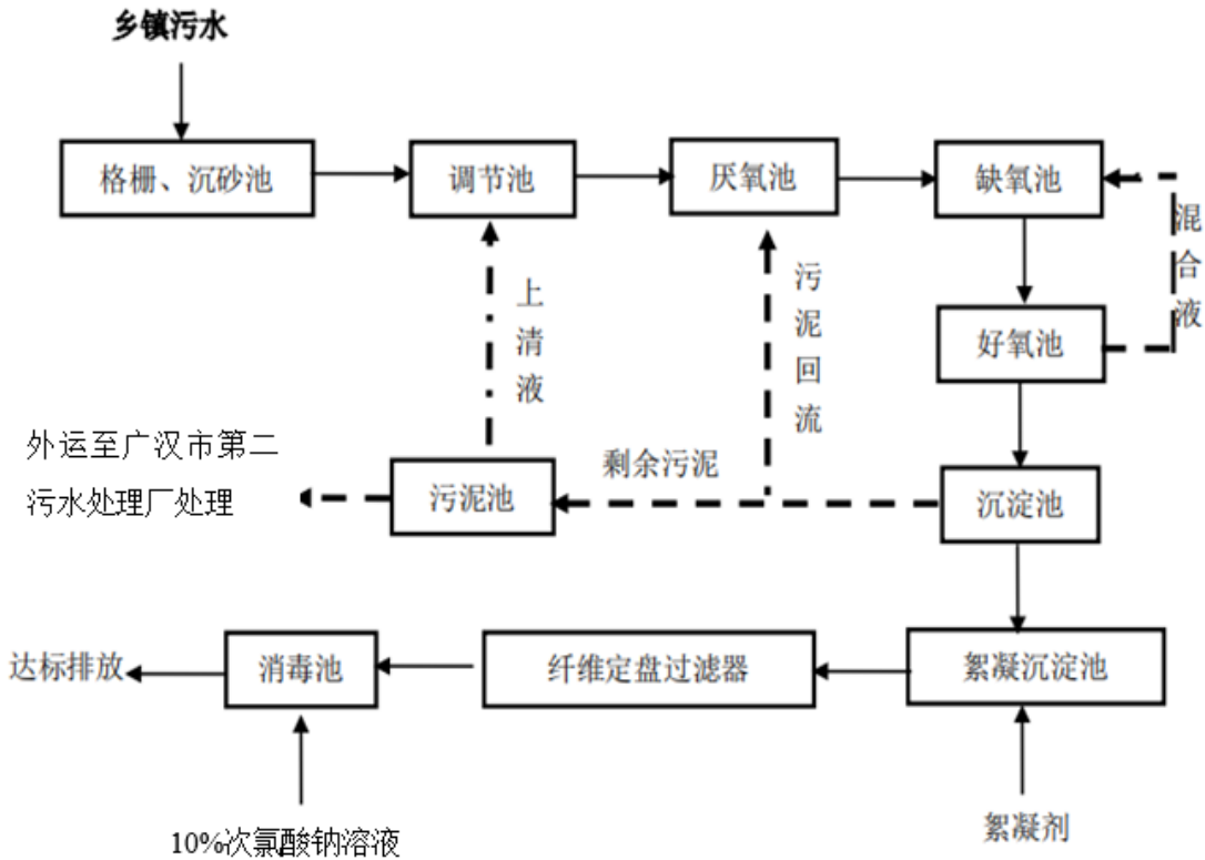
图 2-2 污水处理站工艺流程
