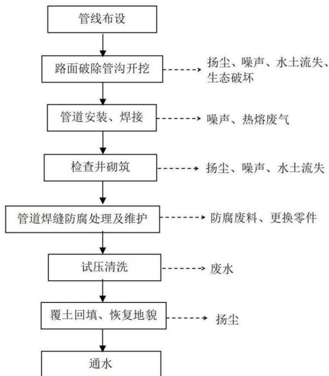
图 4-1 管网施工流程及产污环节图
